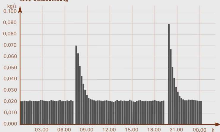
Energieverbrauch – Massenstrom des Kühlmittels ohne Glasabdeckung
