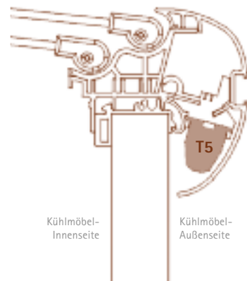
Handlauf mit integriertem Beleuchtungsmodul außen liegend
